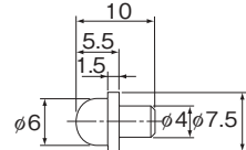
PB1021B形
