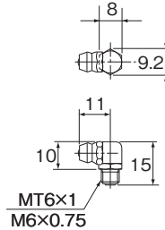
C-MT6×1形 (MT6×1) C-M6F形 (M6×0.75)
