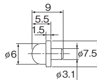
NP3.2×3.5形
