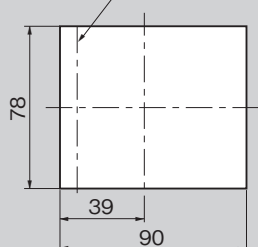
ขนาดการเจาะรูพาดตัวอุปกรณ์ Main body panel drilling dimensions
