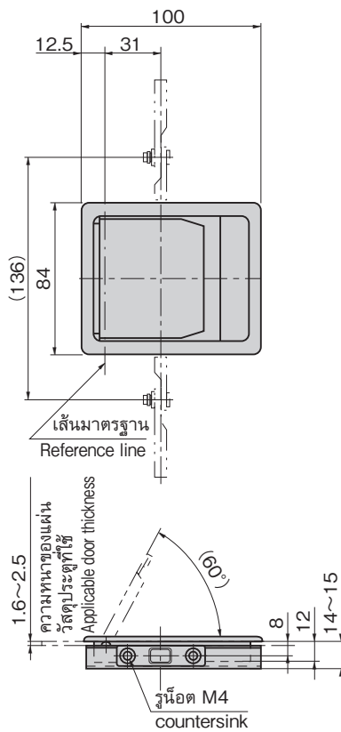
ขนาดการเจาะรูพาดตัวอุปกรณ์ Main body panel drilling dimensions
