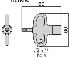
[A-169-H มือจับ] Handle
