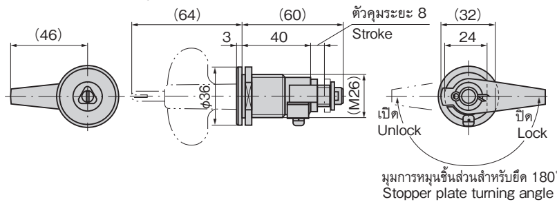
[A-169-1 ตัวอุปกรณ์] Main body
