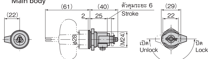
[A-169-H มือจับ] Handle
