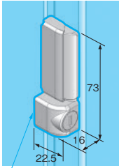
キー付スナップラッチ (標準のスナップラッチを外して交換とします。)
