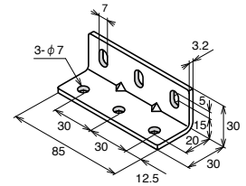
BLSM-3085-6
