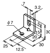
BLSM-3025-6
