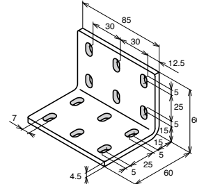
BLHL-8560-6
