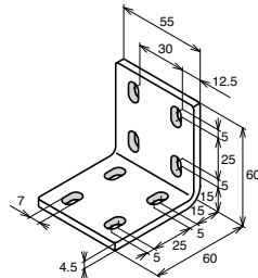
BLHL-5560-6
