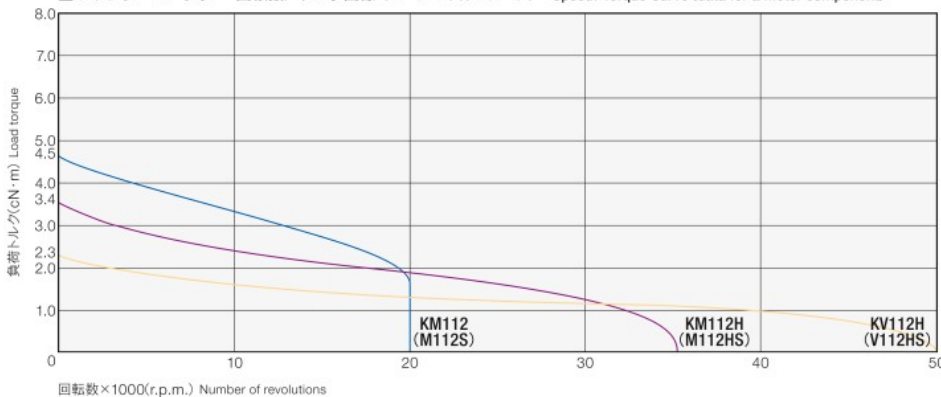
■ スレンダーロータリー 回転数/トルク曲線 (モーター単体のデータ) Speed/Torque Curve (data for a motor component)
