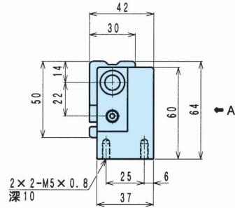
A部矢視図
