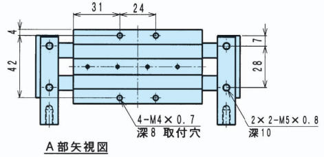
A部矢視図
