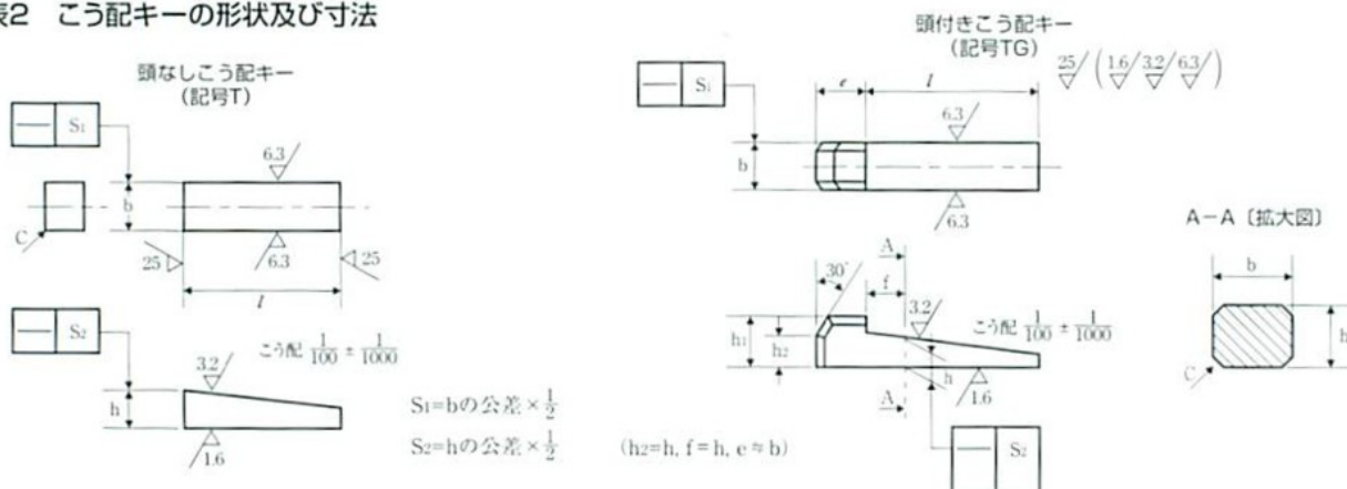
■付表2 こう配キーの形状及び寸法
