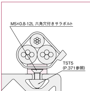
Line8プロファイル T溝への取付。
