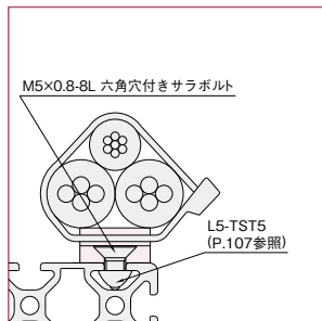
Line5プロファイル T溝への取付。
