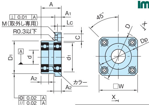
断面 X-X
