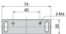
자석브라켓
