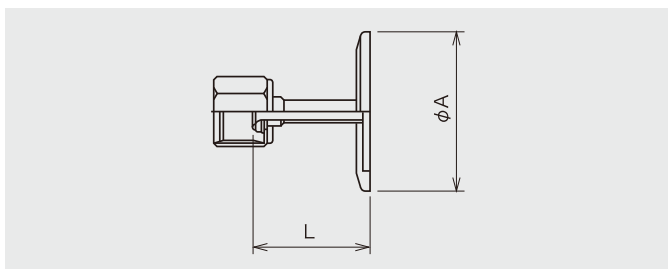
ICF FLANGE+VCR® FEMALE ADAPTOR ICFフランジ+VCR®メスアダプター (Material 材質: VCR®SUS316L ICFフランジSUS304L)
