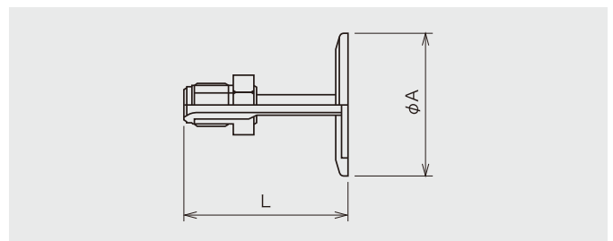
ICF FLANGE+VCR® MALE ADAPTOR ICFフランジ+VCR®オスアダプター (Material 材質: VCR®SUS316L ICFフランジSUS304L)
